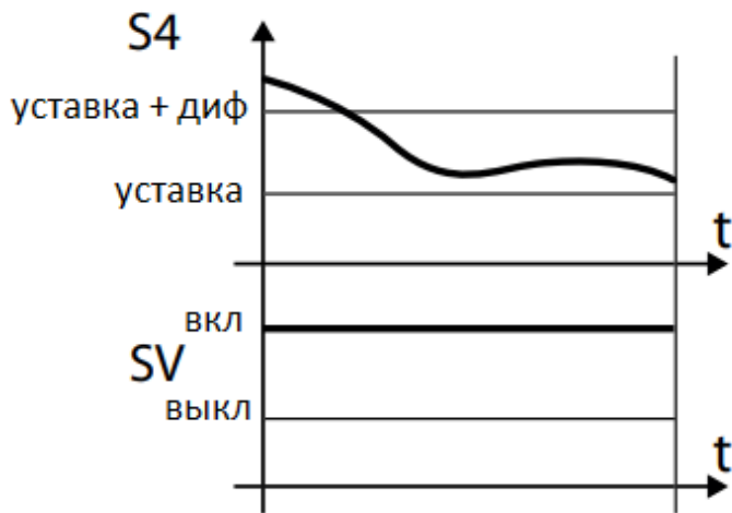
Рис 4.10в Параметры снижения производительности подобраны правильно. Отключение соленоида SV не происходит.
