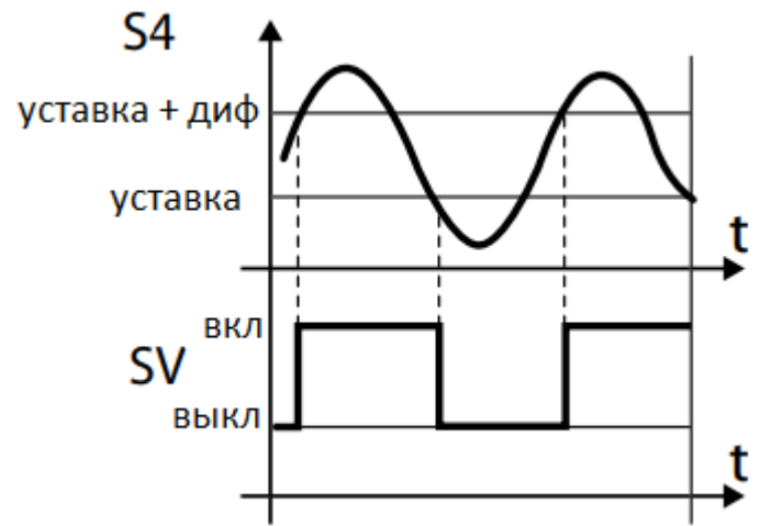
Рис 4.10б Срабатывание соленоидного клапана SV. Смещение уставки перегрева слишком мало. Параметры выбраны некорректно.
