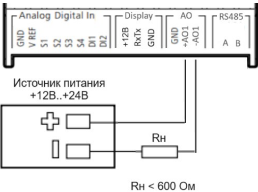
Рис 2.10 Токовая петля аналогового выхода 4-20 мА
