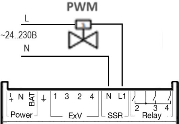
Подключение импульсного клапана к выходу SSR
