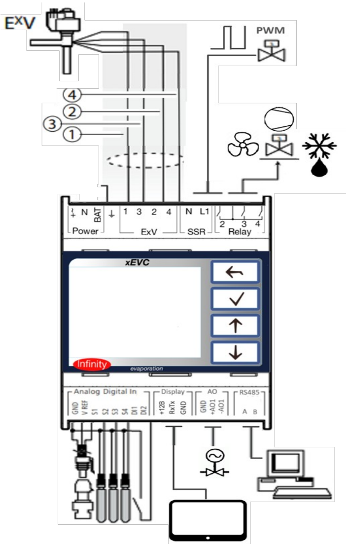
Рис 2.3.1 Схема включения для управления воздушным испарителем
