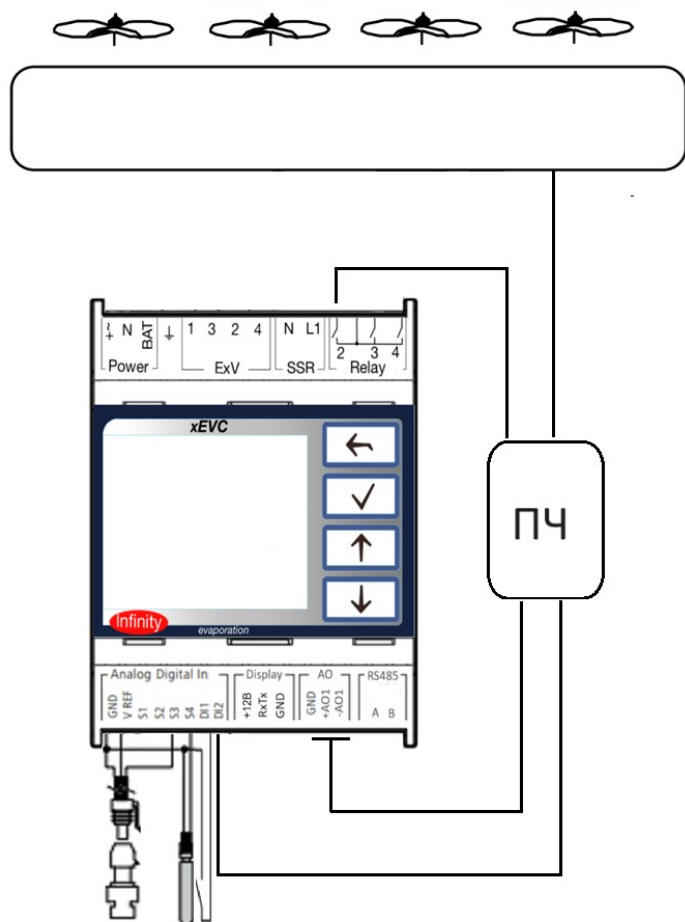
Рис 2.7.1 Схема плавного управления воздушным конденсатором с ПЧ (преобразователем частоты)
