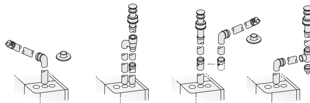
детали и фитинги дымохода EXH*
